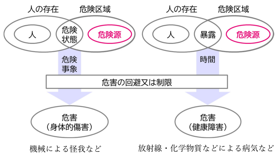
【図 01-10】：危害発生 の条件・流れ（ISO/TR14121-2：2012 より）
